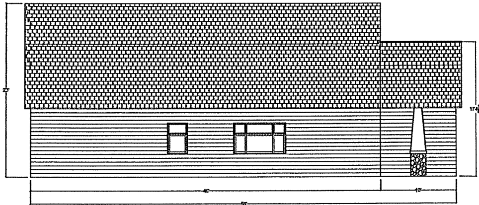
② ELEVATION SCALE: 1/8" = 1'-0"
