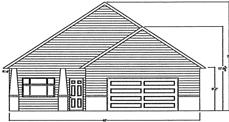
① ELEVATION SCALE: 1/8" = 1'-0"
