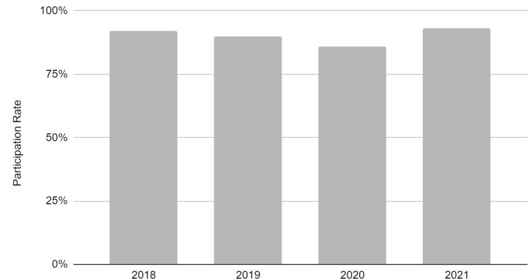
Participation Rate
