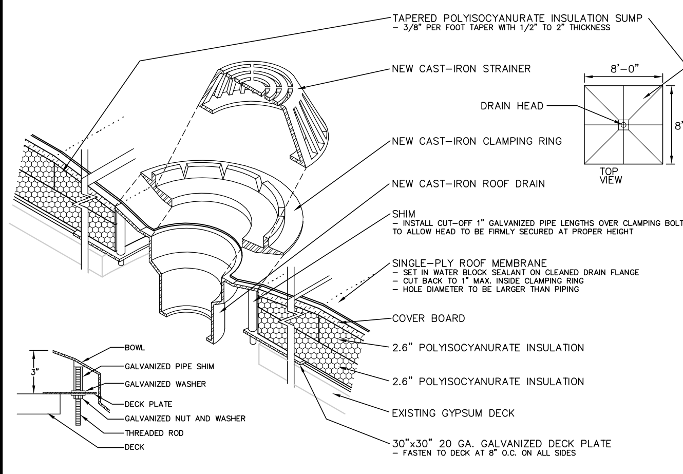
6 DRAINING FLASHING N.T.S.
