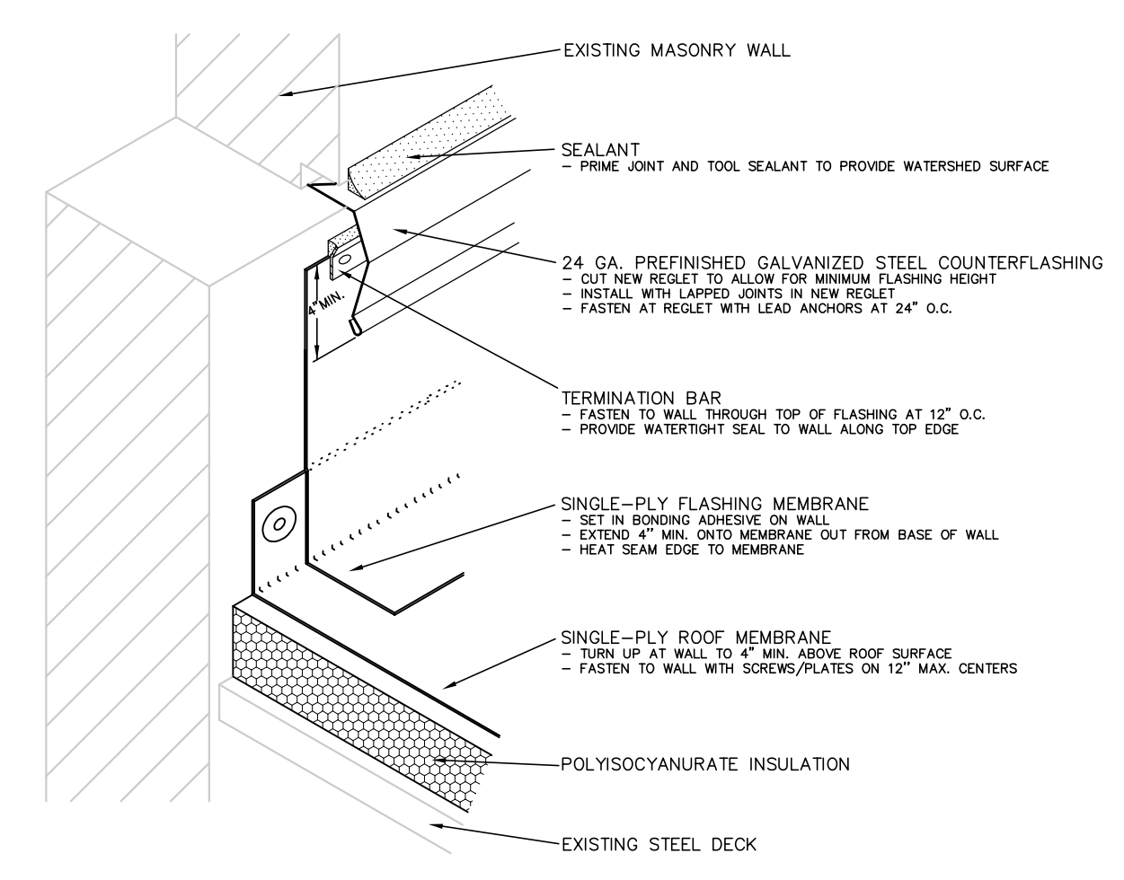
2 WALL FLASHING N.T.S.
