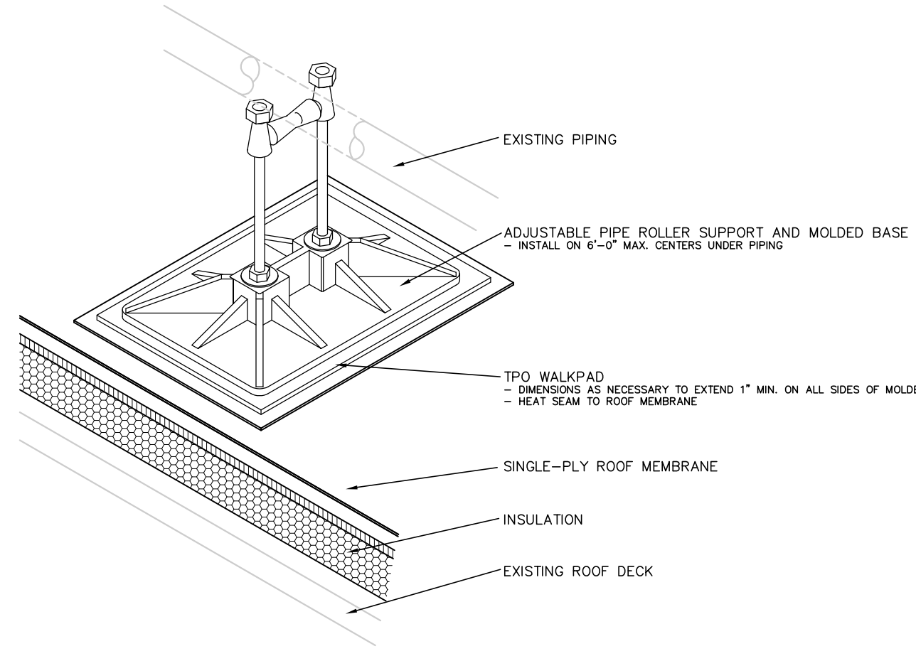
8 PIPE ROLLER SUPPORT N.T.S.
