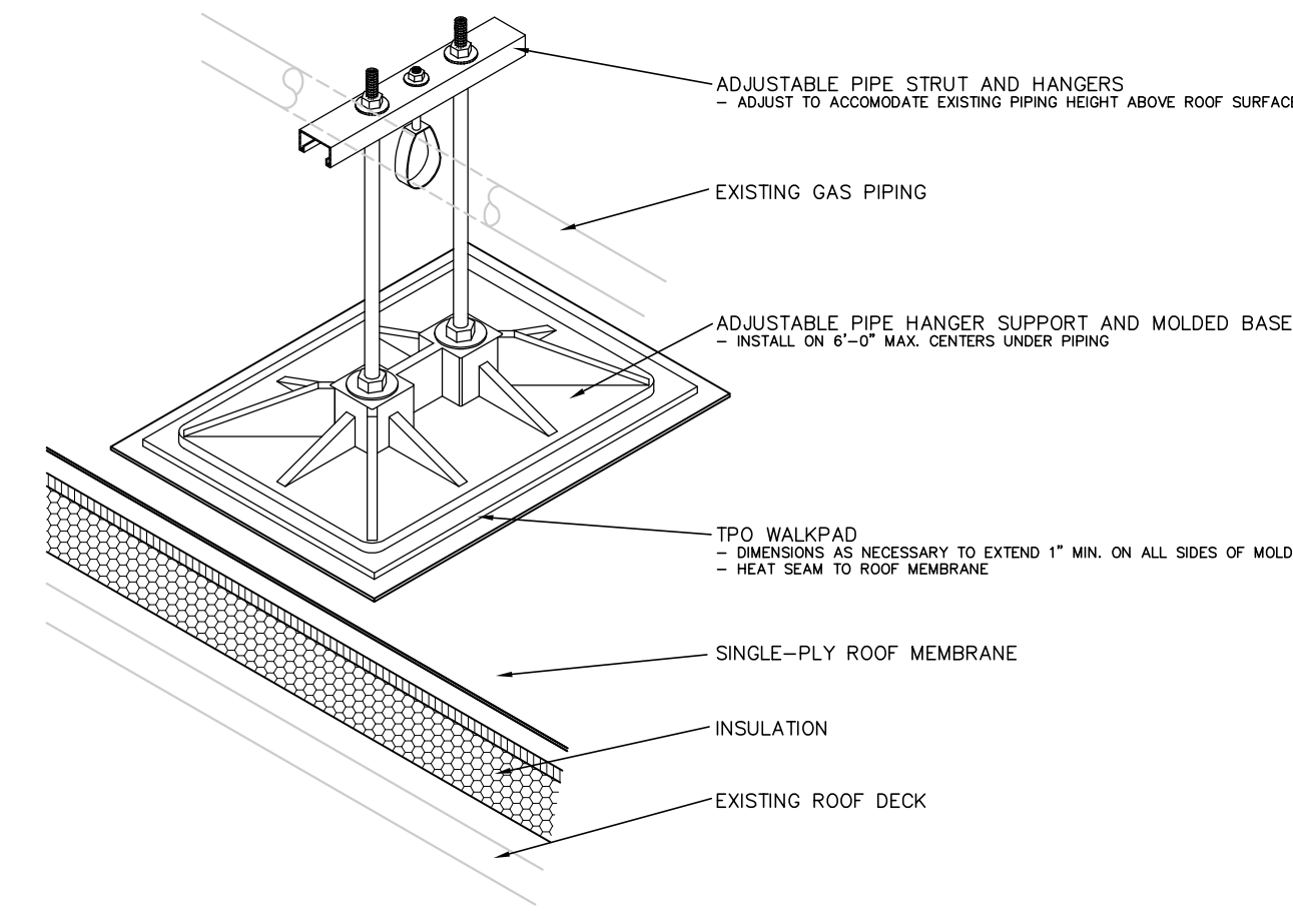
9 PIPE HANGER SUPPORT N.T.S.
