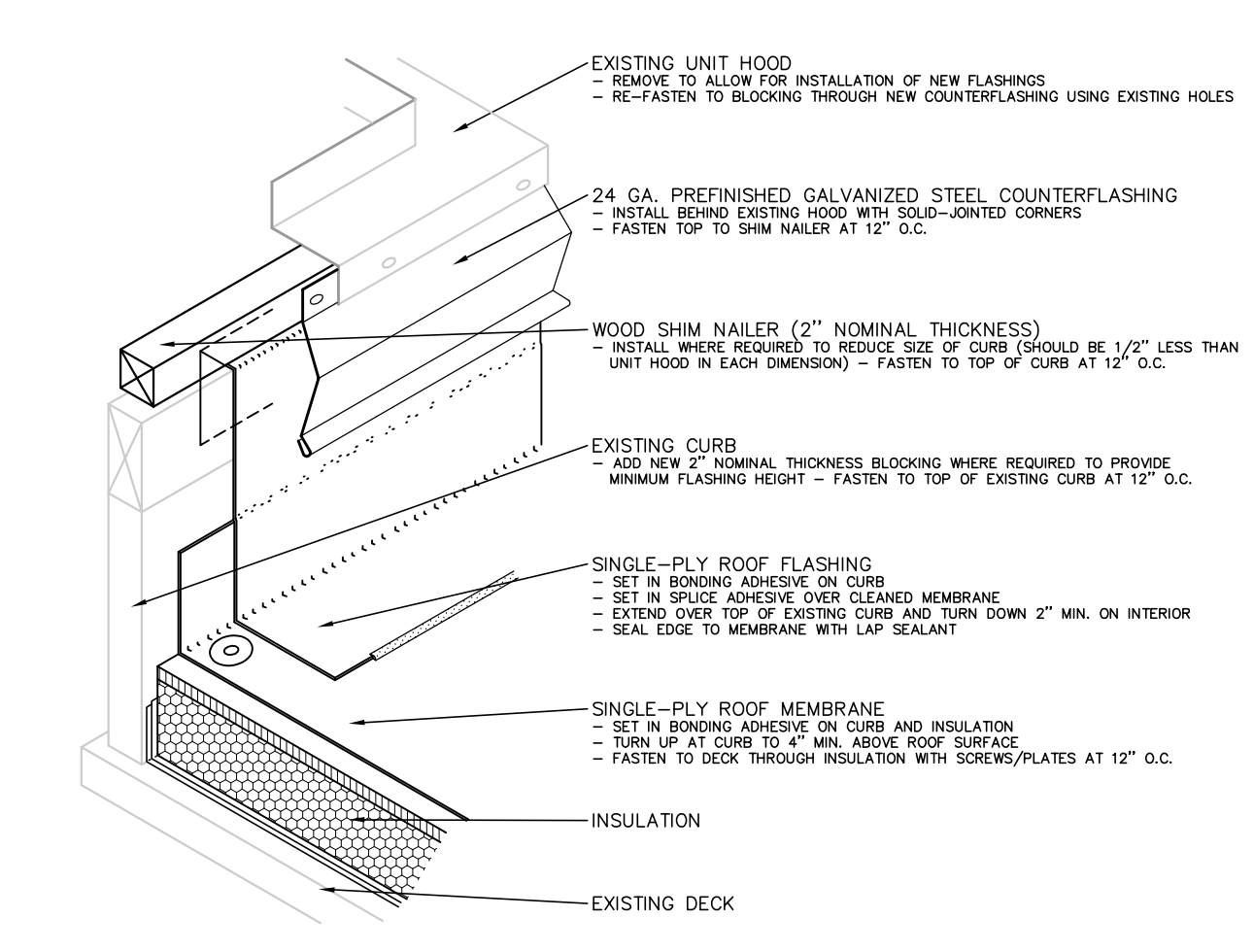
4 EXHAUST FAN CURB N.T.S.
