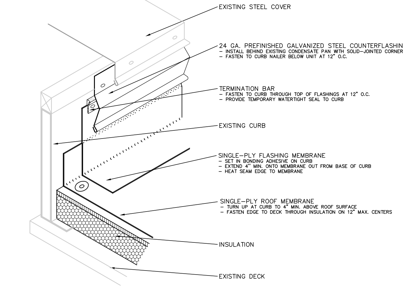
10 ROOF TOP UNIT CURB FLASHING N.T.S.
