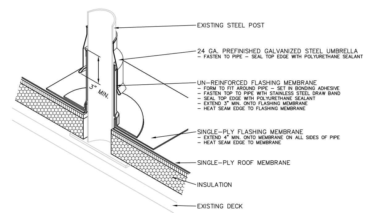
7 STEEL POST FLASHING N.T.S.
