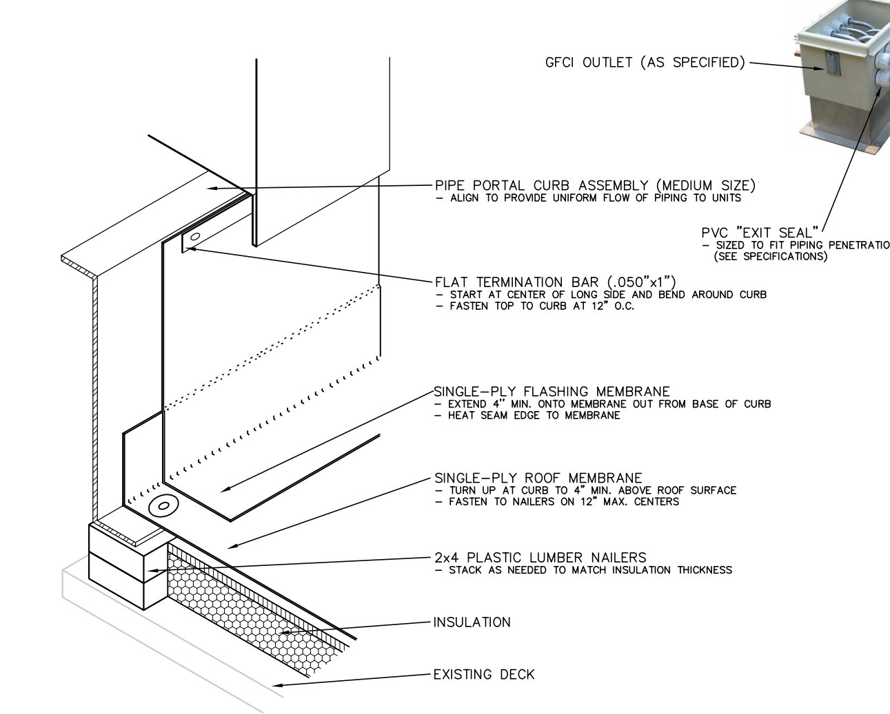
5 SMART BOX FLASHING N.T.S.
